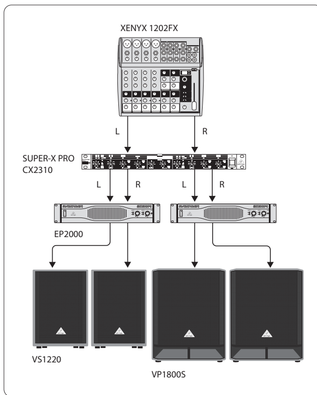
Fig. 5.3: Tweeweg stereobediening met subwoofers
