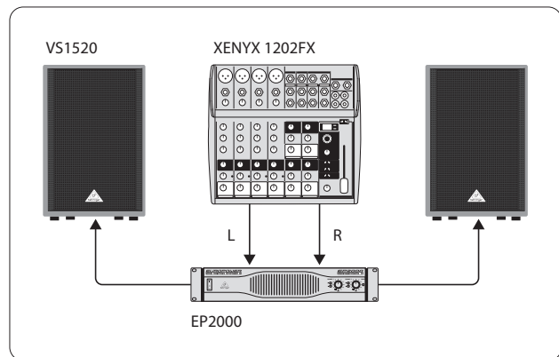
Abb. 5.1: Breitbandiger Stereobetrieb
